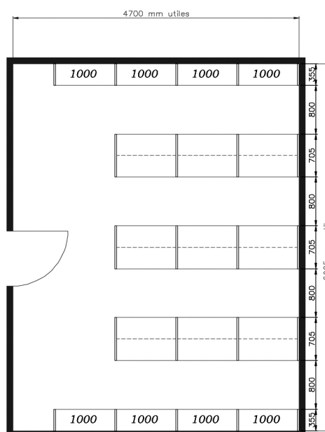
RAYONNAGE FIXE (156 ml de tablette)
