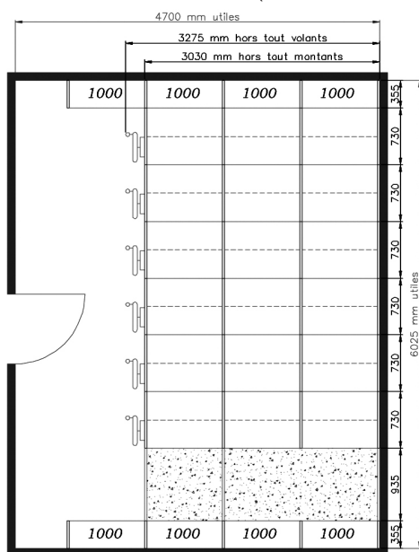
RAYONNAGE MOBILE (264 ml de tablette)
